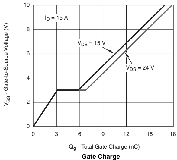
I_D = 15\text{ A} V_{DS} = 15\text{ V} V_{DS} = 24\text{ V} Gate Charge
